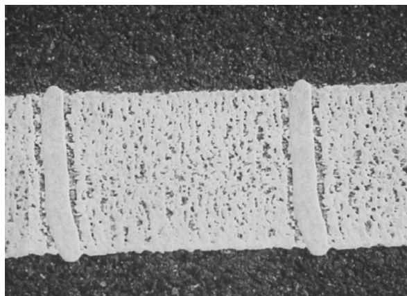
Obr. 7: Příklad rozmístění jednotlivých baretů, vzhled struktury VDZ
