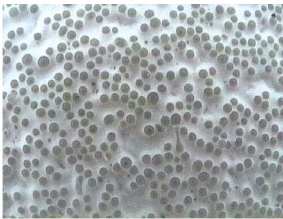
Obr. 12: Příklad optimálního zabudování balotiny do hmoty
