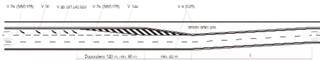
Obrázek 29: Příklad VDZ snížení počtu jízdních pruhů s ukončením levého jízdního pruhu
