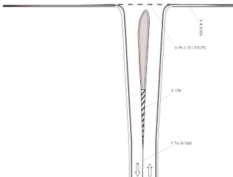
Obrázek 40: Příklad VDZ kapkovitého dopravního ostrůvku.
