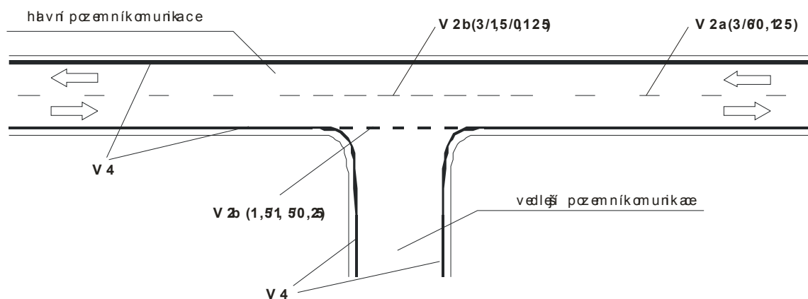
Obrázek 15a: Příklad VDZ v oblasti křižovatky - dovolené předjíždění na hlavní pozemní komunikaci
