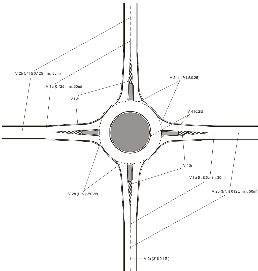
Obrázek 20a: Příklad VDZ na okružní křižovatce
