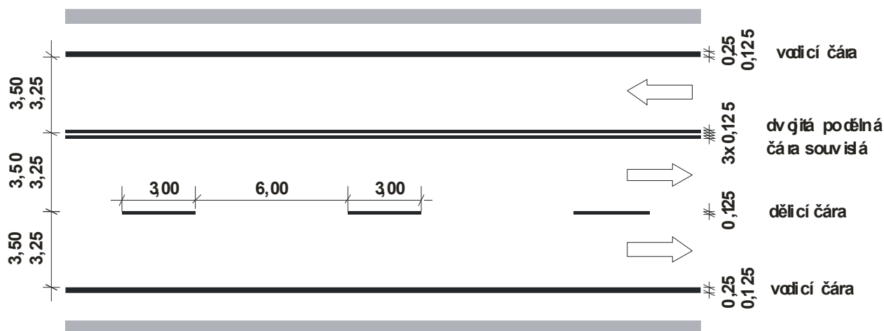
Obrázek 4: Příklad VDZ na pozemní komunikaci s vozovkou se třemi jízdními pruhy
