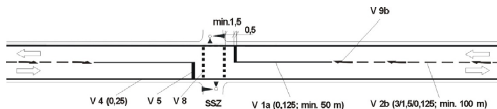
Obrázek 36: Příklad VDZ přejezdu pro cyklisty řízeného SSZ
