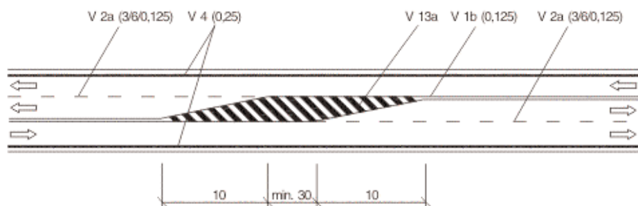
Obrázek 24: Příklad VDZ zvýšení počtu jízdních pruhů
