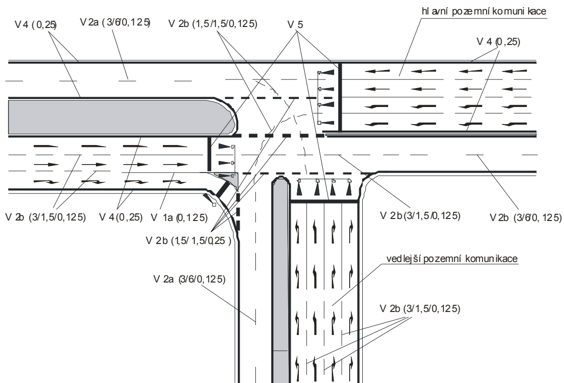
Obrázek 19: Příklad VDZ na křižovatce řízené SSZ
