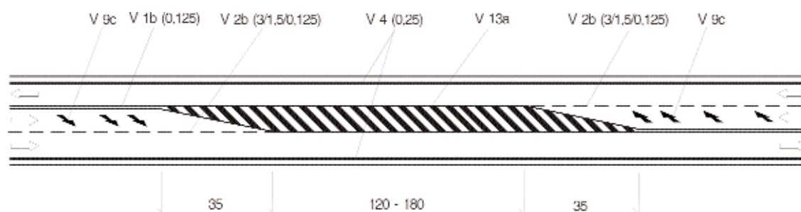
Obrázek 23: Příklad zvýšení počtu jízdních pruhů - detail VDZ
