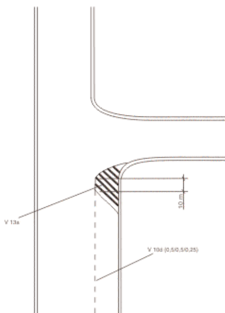
Obrázek 14: Příklad VDZ parkovacího pruhu.
