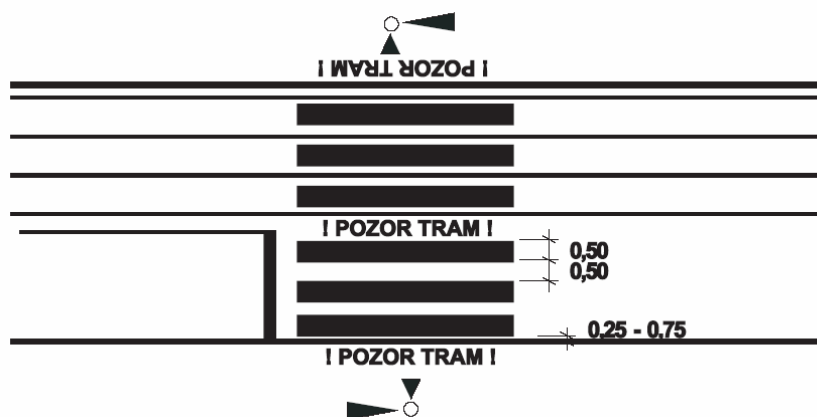
Obrázek 33b: Příklad VDZ přechodu pro chodce na pozemní komunikaci s tramvajovým pásem v úrovni vozovky se SSZ
