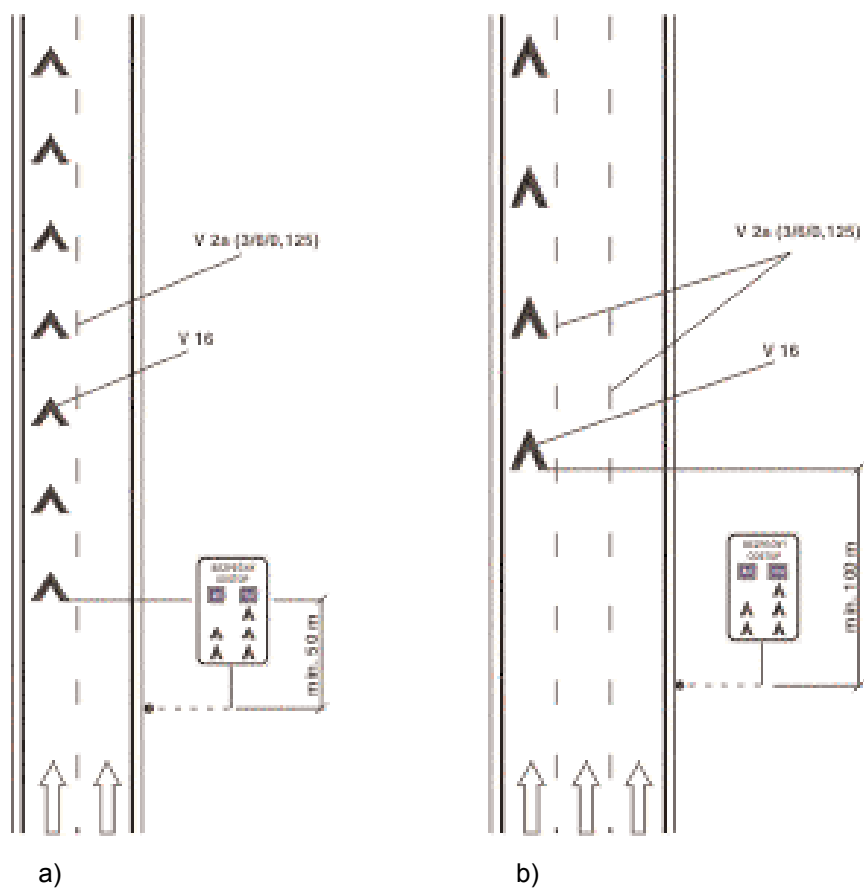
Obrázek 45: Příklad provedení značky č. V 16
