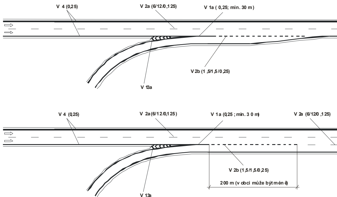
Obrázek 9: Příklady VZD připojovacího pruhu
