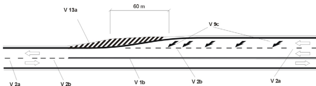
Obrázek 25: Příklad VDZ snížení počtu jízdních pruhů mimo dálnice (levý pruh průběžný), ukončení jízdního pruhu může být zdůrazněno užitím značky č. V 9c
