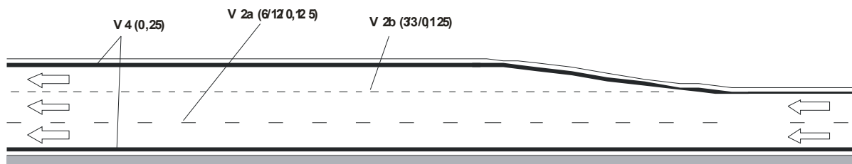
Obrázek 11b: Příklad VDZ jízdního pruhu pro pomalá vozidla s možností předjíždění.
