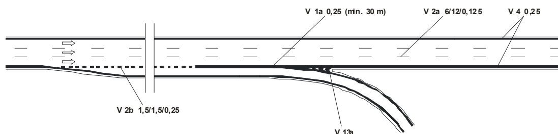
Obrázek 8: Příklad VDZ odbočovacího pruhu
