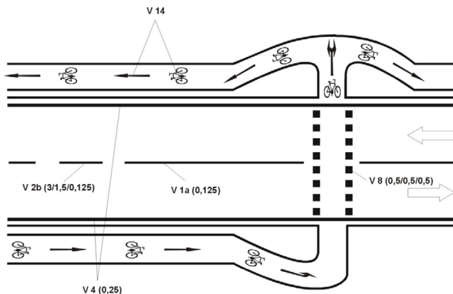
Obrázek 34: VDZ přejezdu pro cyklisty
