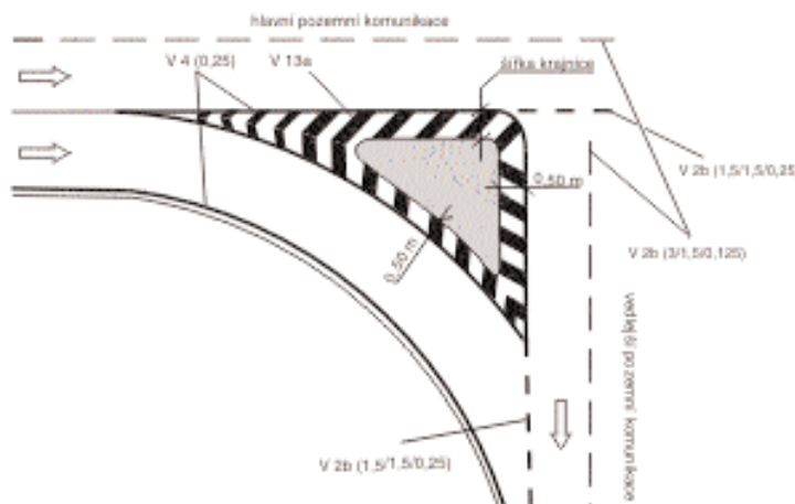
Obrázek 41: Příklad VDZ směrovacího dopravního ostrůvku
