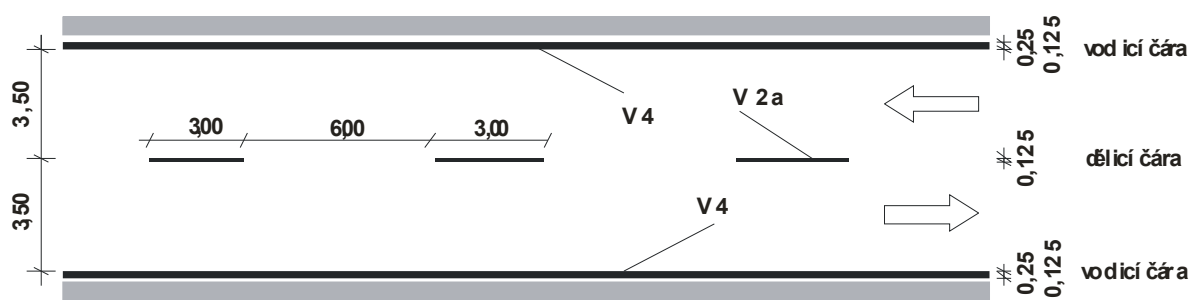
Obrázek 3: Příklad VDZ na pozemní komunikaci kategorie S 9,5 MS, MO 14
