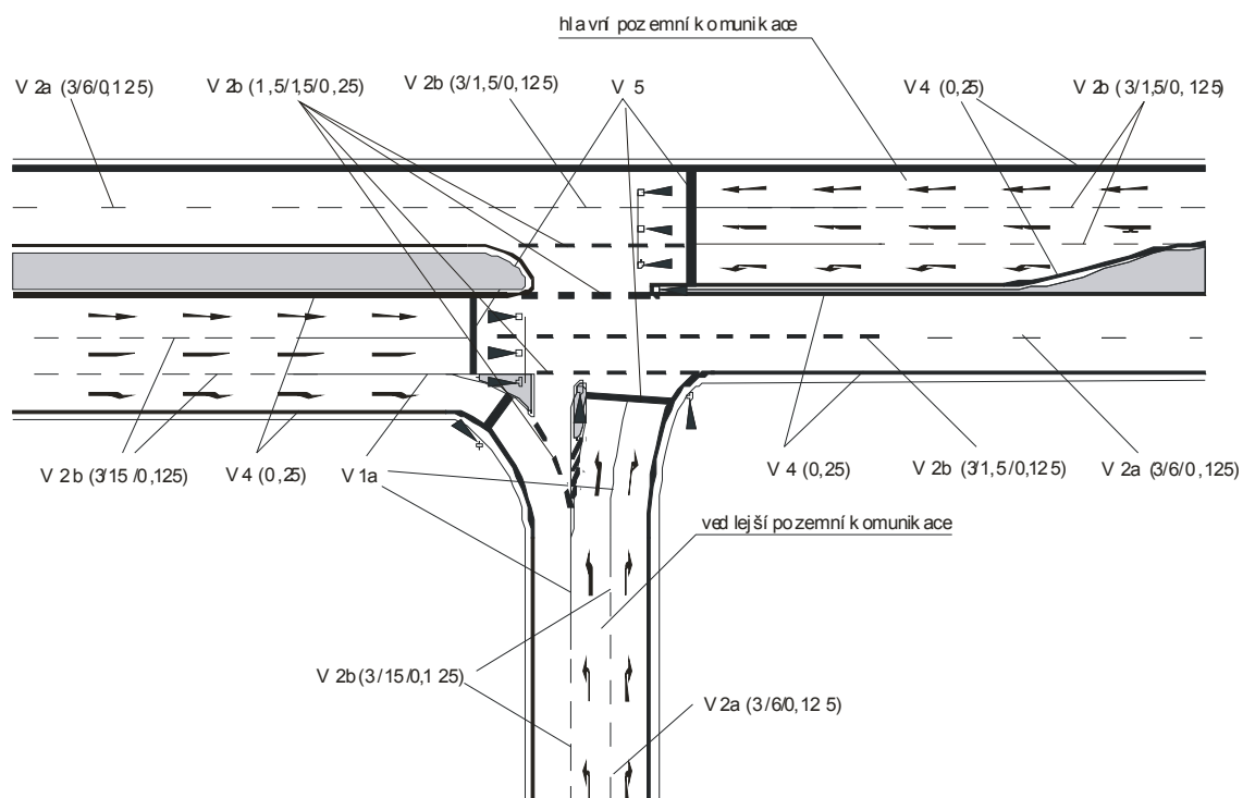
Obrázek 18: Příklad VDZ na křižovatce řízené SSZ
