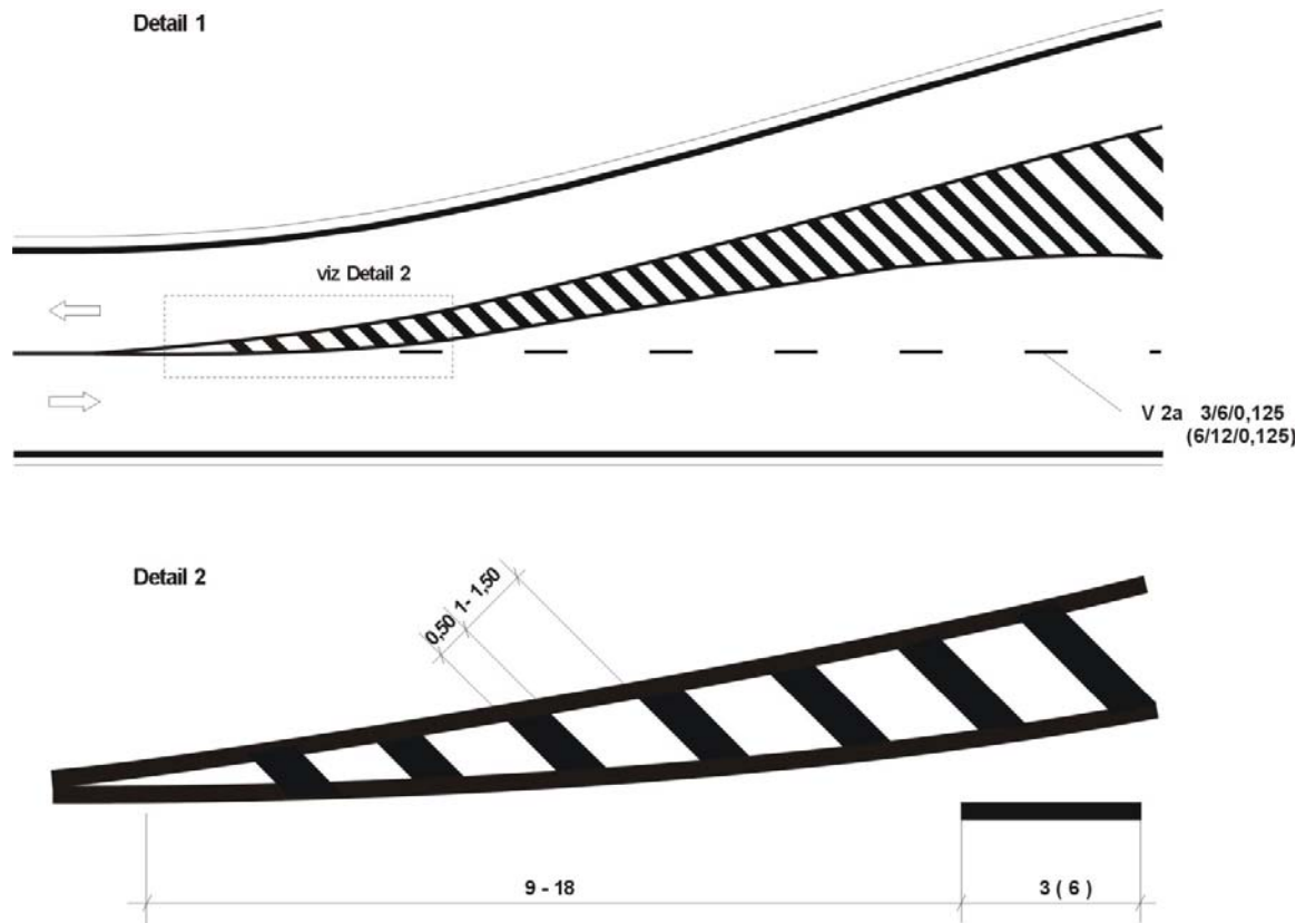
Obrázek 30: Příklad VDZ jízdních pruhů - přechod čtyřpruhové směrově rozdělené pozemní komunikace do dvoupruhové směrově nerozdělené pozemní komunikace.
