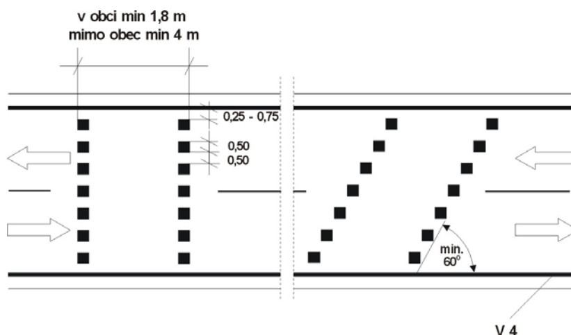
Obrázek 34: VDZ přejezdu pro cyklisty
