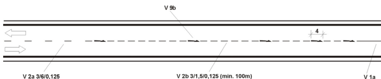
Obrázek 37: Příklad užití a umístění předběžných šípek č. V 9b
