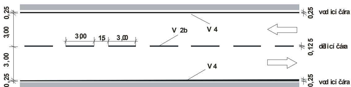
Obrázek 2: Příklad VDZ na pozemní komunikaci s vozovkou o šířce od 6 m do 7,00 m
