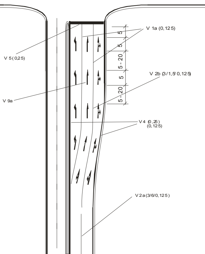
Obrázek 7: Příklad VDZ řadicích pruhů
