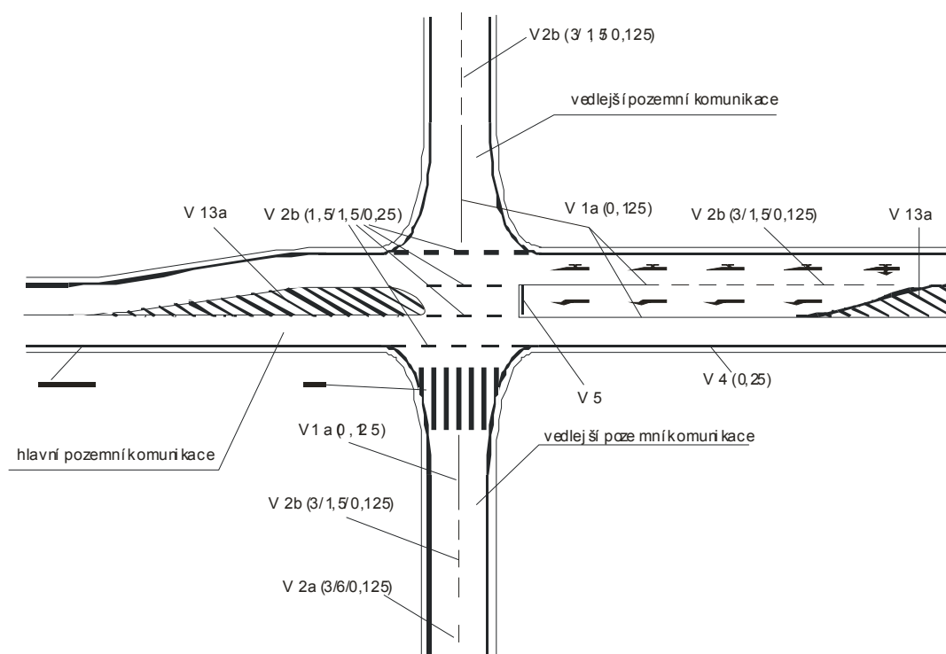
Obrázek 17b: Příklad VDZ na křižovatce s řadícími pruhy bez zvýšeného ostrůvku na hlavní pozemní komunikaci
