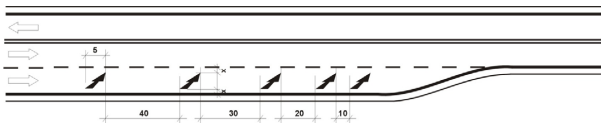
Obrázek 38: Příklad užití a umístění předběžných šípek č. V 9c (mimo obec)
