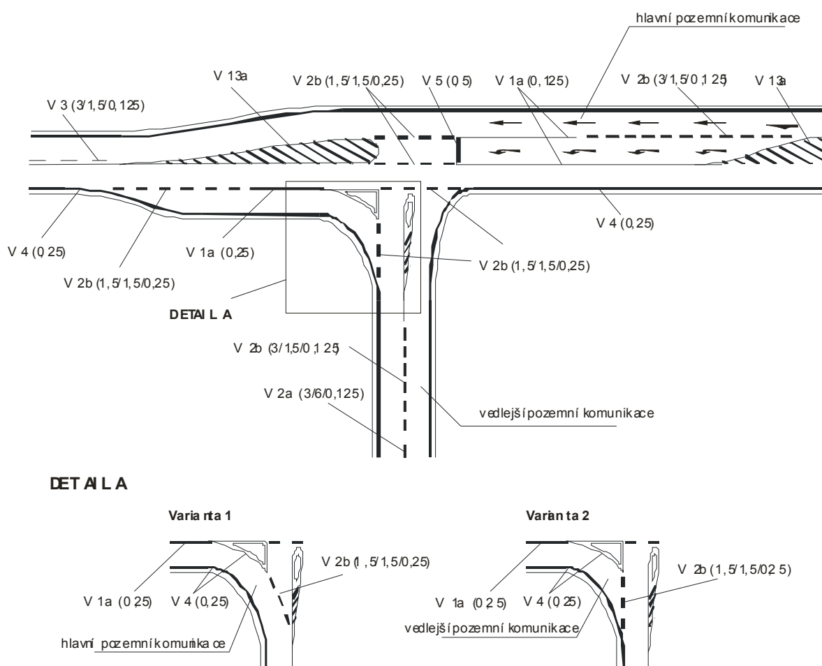
Obrázek 16: Příklad VZD na křižovatce s řadícími pruhy a odbočovacími pruhy na hlavní pozemní komunikaci
