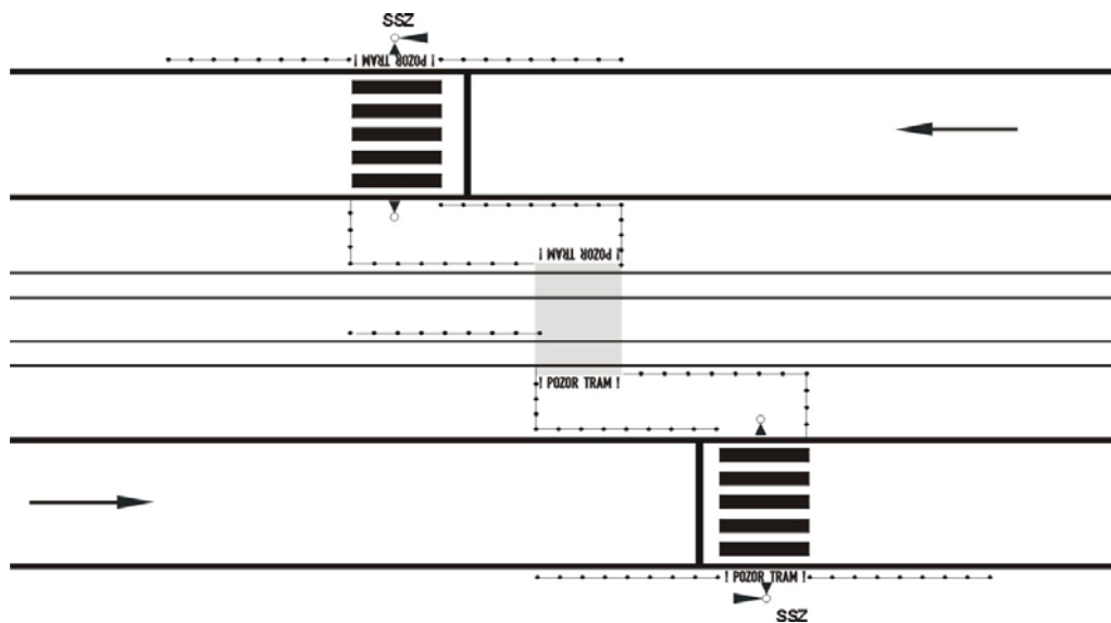
Obrázek 33c: Příklad VDZ přechodu pro chodce na pozemní komunikaci se zvýšeným tramvajovým pásem se SSZ
