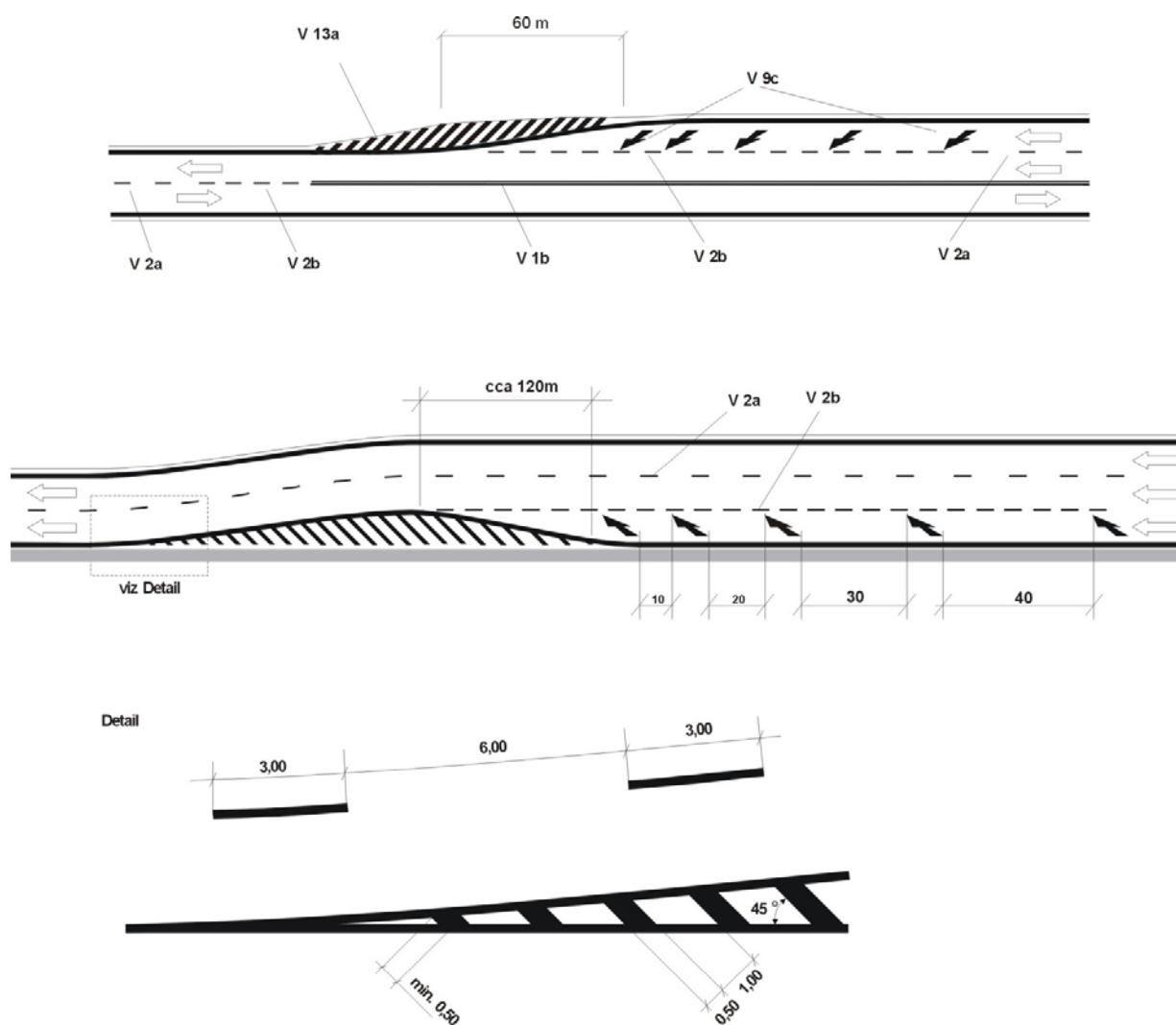
Obrázek 26: Příklad VDZ snížení počtu jízdních pruhů s ukončením levého jízdního pruhu (stavební ukončení pravého jízdního pruhu)
