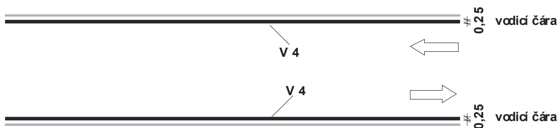
Obrázek 1: Příklad VDZ na pozemní komunikaci s vozovkou o šířce menší než 6 m
