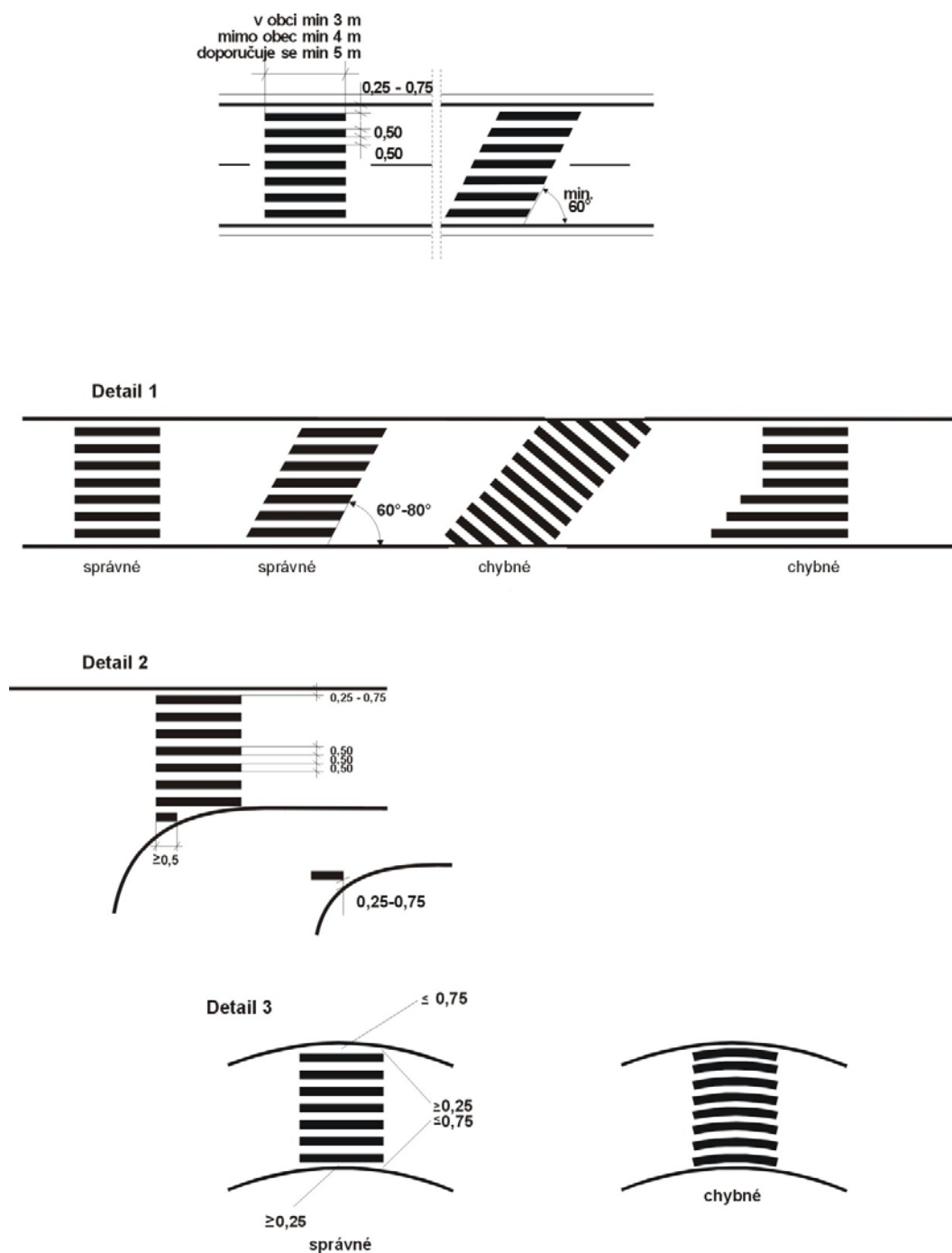
Obrázek 32: Detaily VDZ přechodu pro chodce
