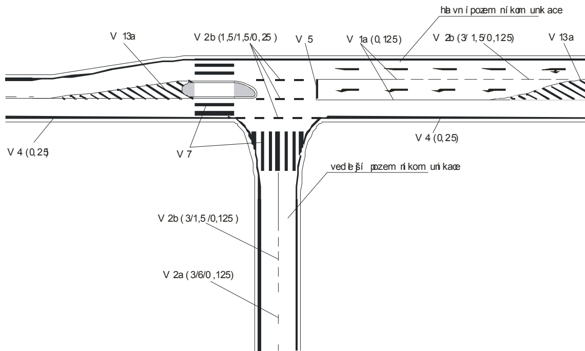
Obrázek 17a: Příklad VDZ na křižovatce s řadicími pruhy s ochranným zvýšeným ostrůvkem na hlavní pozemní komunikaci
