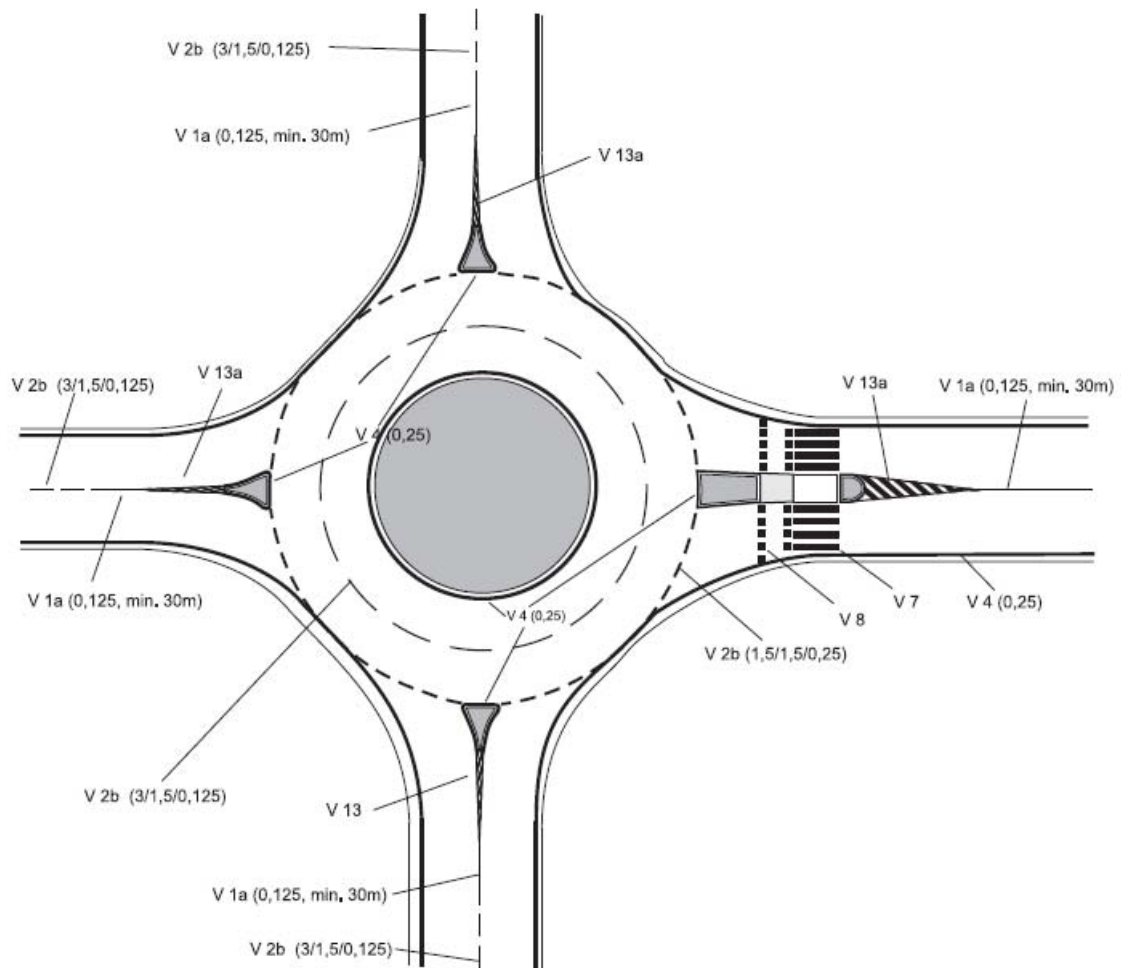
Obrázek 20b: Příklad VDZ na okružní křižovatce
