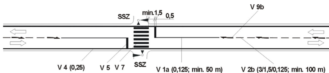
Obrázek 33a: Příklad VDZ přechodu pro chodce se SSZ
