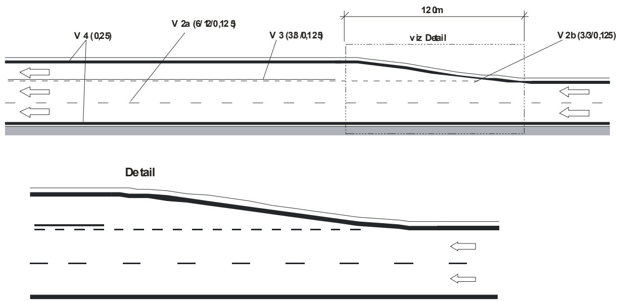
Obrázek 11a: Příklad VDZ jízdního pruhu pro pomalá vozidla.
