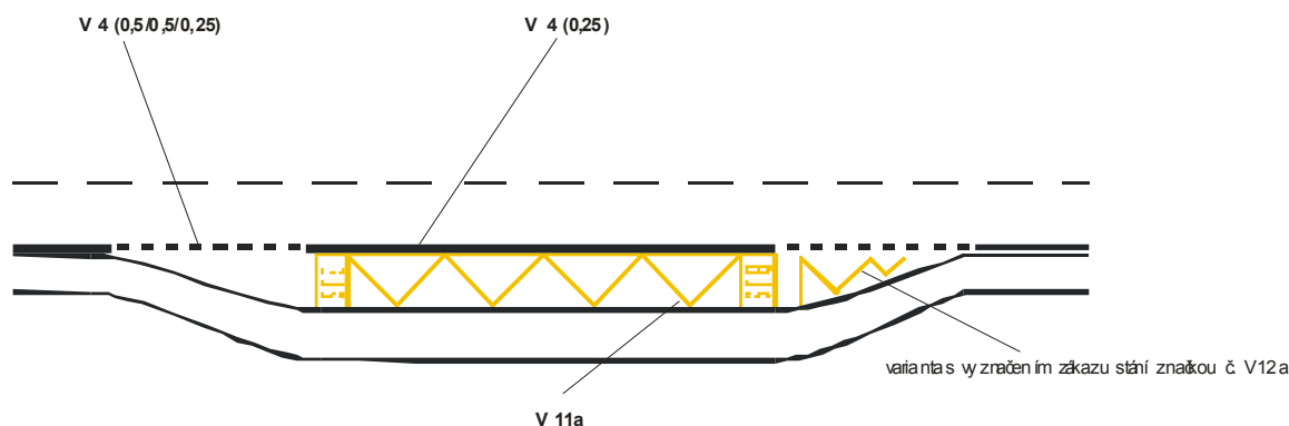
Obrázek 13: Příklad VDZ zastávkového pruhu s vyznačením zastávky.
