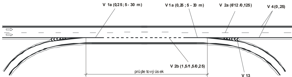
Obrázek 10: Příklad VZD průpletového úseku
