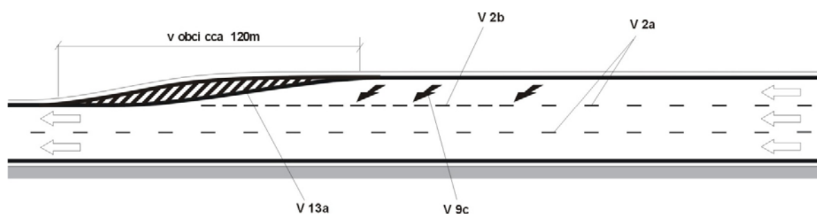
Obrázek 27: Příklad VDZ snížení počtu jízdních pruhů s ukončením pravého jízdního pruhu (stavební ukončení pravého jízdního pruhu)
