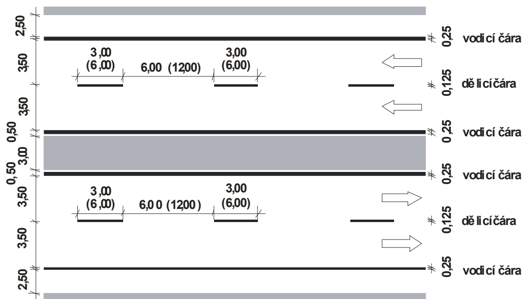
Obrázek 6: Příklad VDZ směrově rozdělené pozemní komunikace kategorie S 24,5
