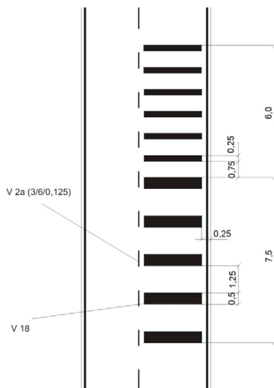
Obrázek 46b: Příklad provedení značky č. V 18. Opticko-psychologická brzda
