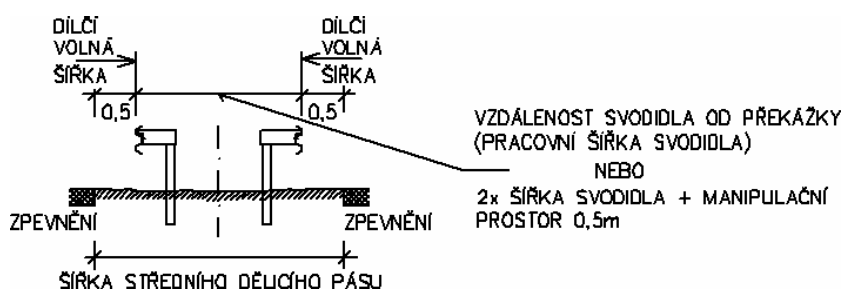
Obrázek 1 – Stanovení minimální šířky středního dělicího pásu pro dvě souběžná ocelová svodidla
