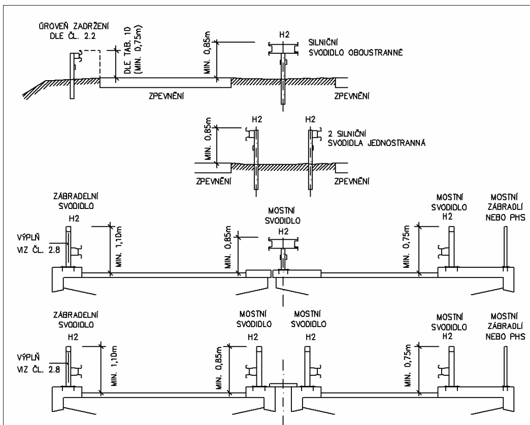
Obrázek 3 – Příklad silničního, mostního a zábradelního svodidla, pokud má být v SDP svodidlo úrovně zadržetí H2
