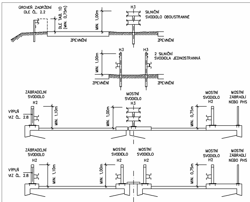
Obrázek 2 – Příklad silničního, mostního a zábradelního svodidla, pokud má být v SDP svodidlo úroveň zadržení H3
