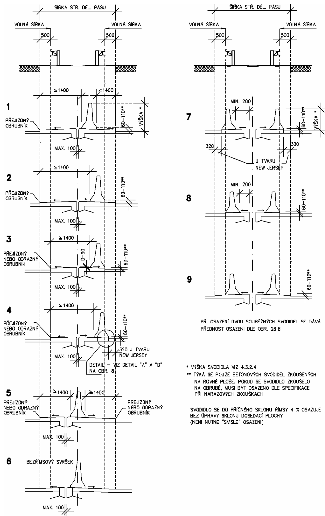
Obrázek 26 - Betonové svodidlo tvaru New Jersey a tvarů velmi podobných ve středním dělicím pásu
