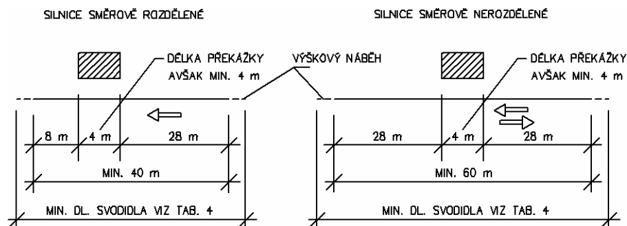
Obrázek 13 - Svodidlo před překážkou a místem nebezpečí
