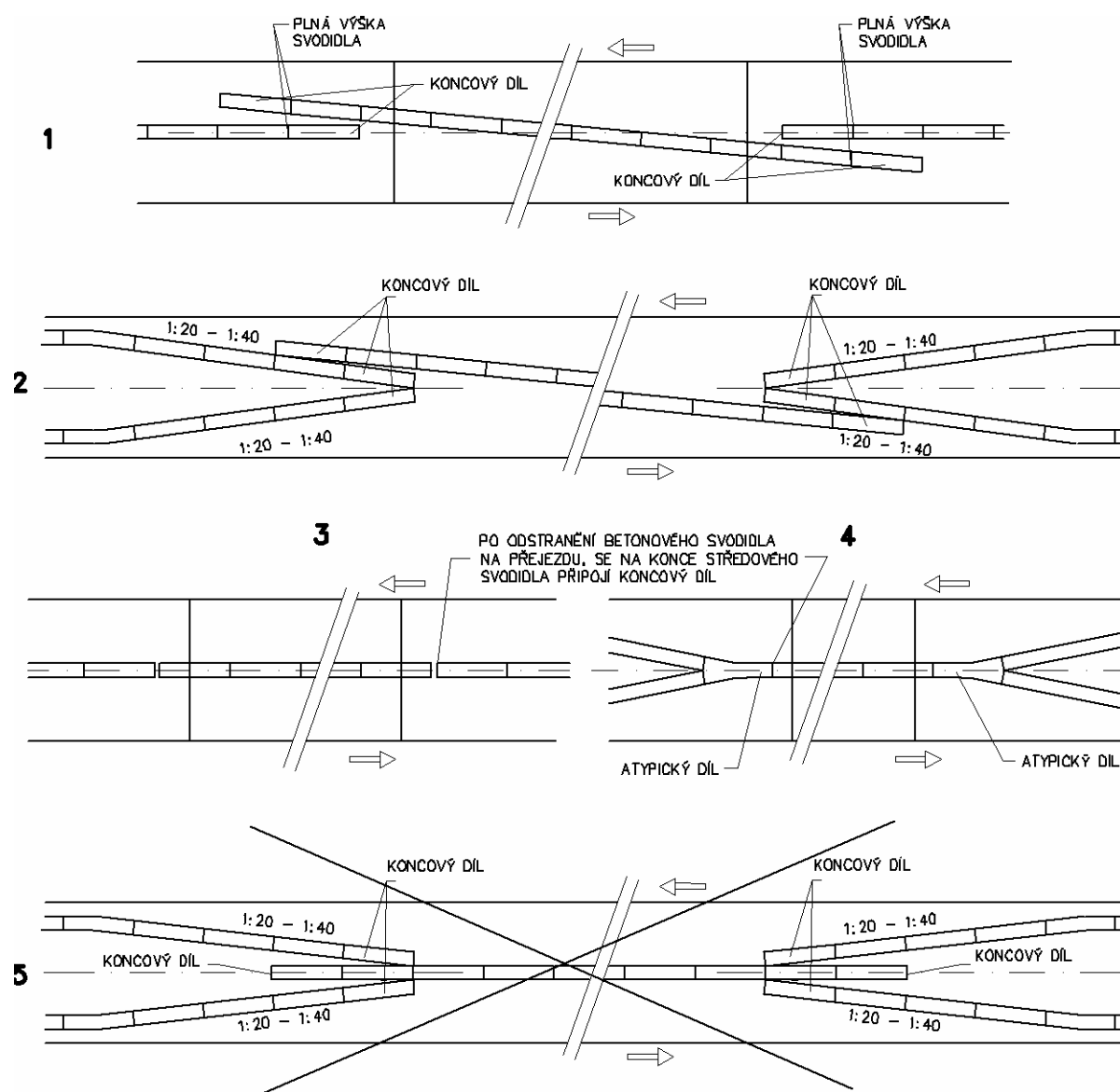
Obrázek 23 - Betonové svodidlo na přejezdech středních dělicích pásů
