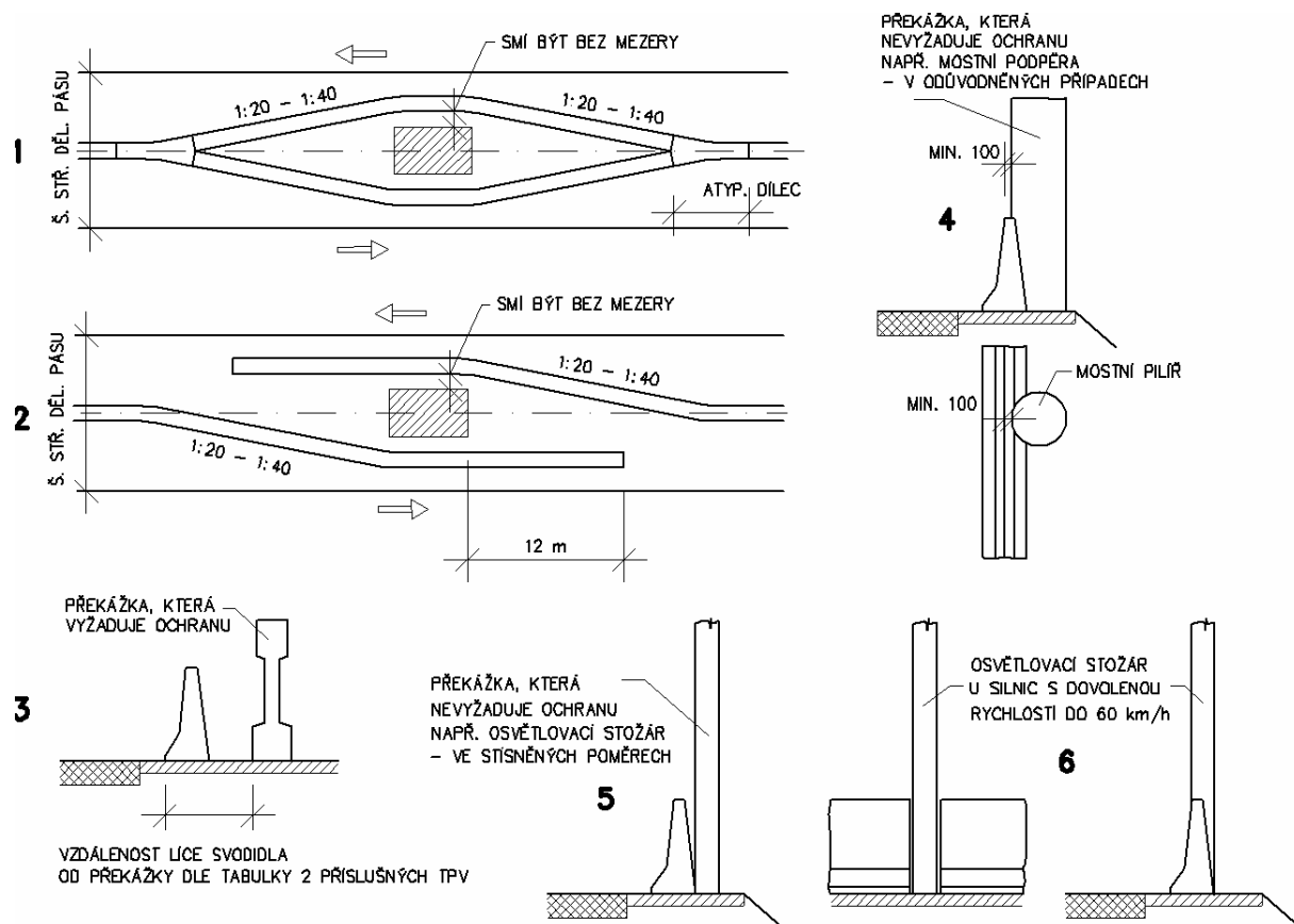
Obrázek 16 - Vzdálenost betonového svodidla od překážky
