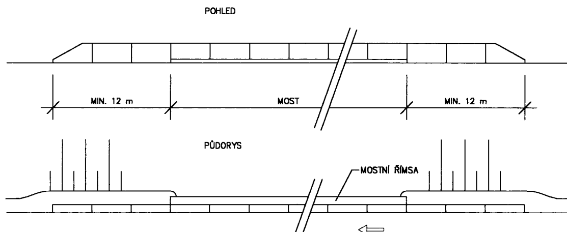
Obrázek 28 - Svodidlo nepokračuje mimo most
