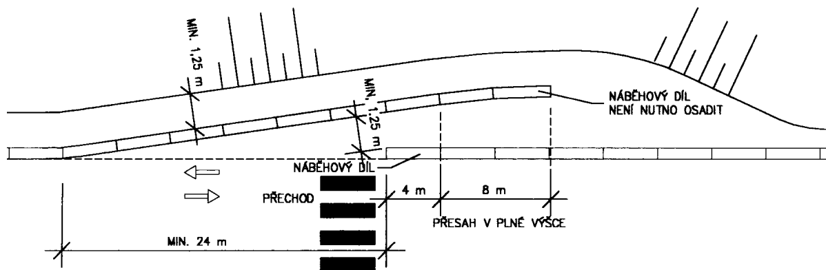
Obrázek 21 - Přerušení betonového svodidla - přechod pro chodce
