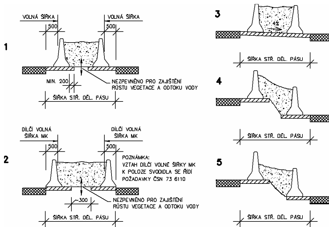
Obrázek 12 - Dvě betonová svodidla se zásepem ve středním dělicím pásu
