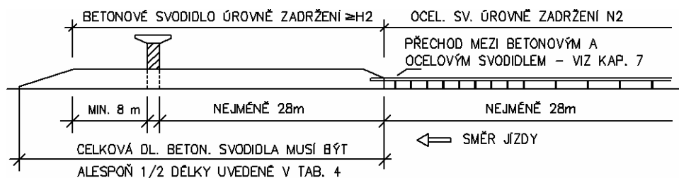
Obrázek 14 – Příklad vložení betonového svodidla do svodidla úr. zadržení N2 před mostním pilířem
