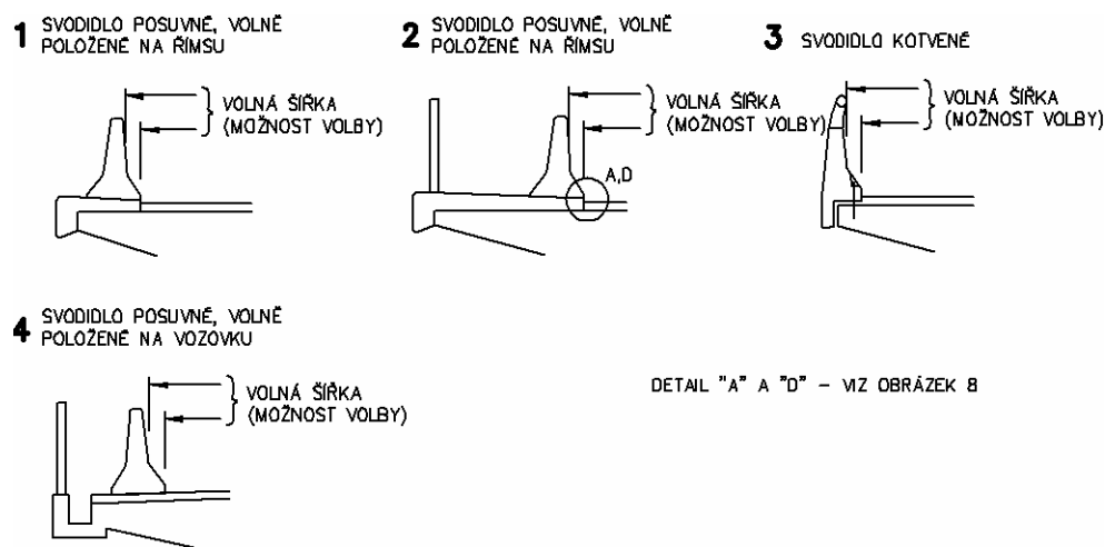
Obrázek 25 - Betonové svodidlo na okraji mostu - nejčastěji používaná řešení
