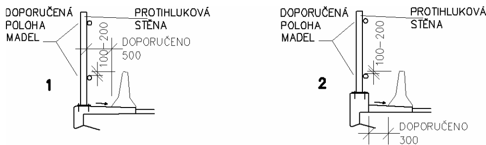
Obrázek 27 - Betonové svodidlo u protihlukové stěny
