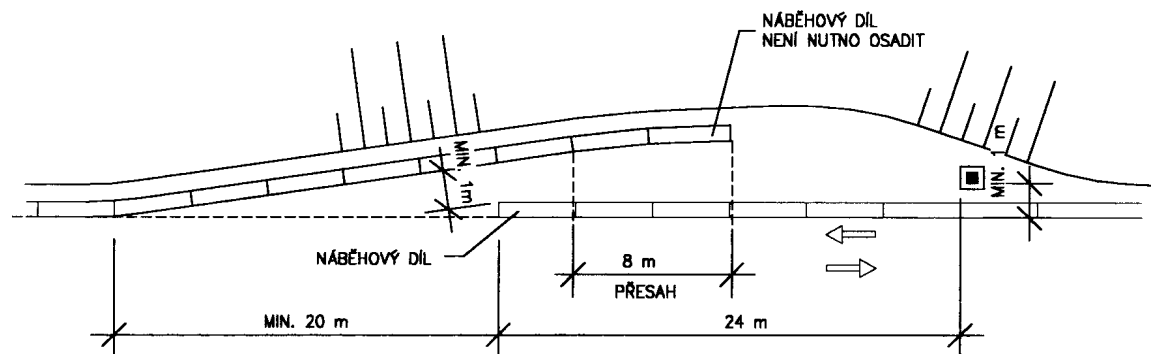
Obrázek 20 - Betonové svodidlo u tíšňové hlásky - silnice směrově nerozdělené
