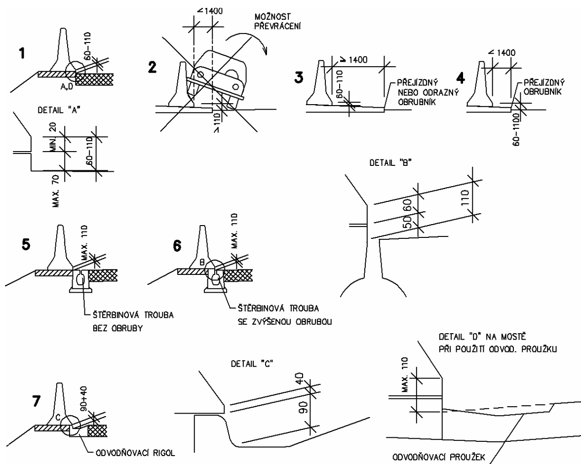
Obrázek 8 – Osazení svodidla tvaru New Jersey na zvýšenou obrubu
