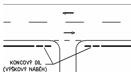
Obrázek 22 – Betonové svodidlo u připojení, sjezdů a křižovatek
