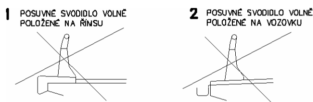
Obrázek 24 - Betonové svodidlo na okraji mostu – řešení dovolené pouze za podmínek uvedených v 6.1.1
