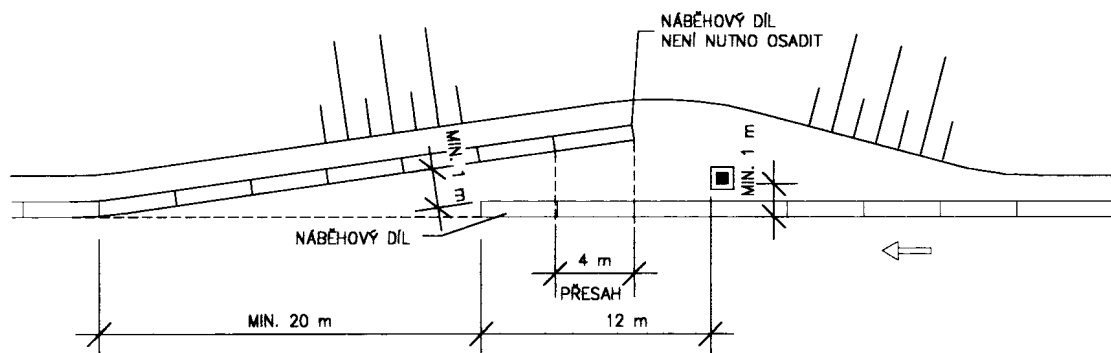
Obrázek 19 - Betonové svodidlo u tísňové hlásky - silnice směrově rozdělené
