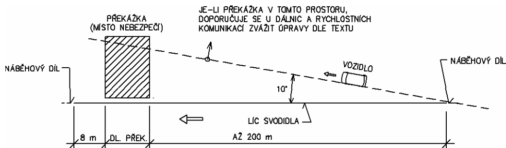
Obrázek 15 - Nebezpečí nárazu vozidla do překážky vyjetím z vozovky před svodidlem, je-li za svodidlem zpevněná plocha
