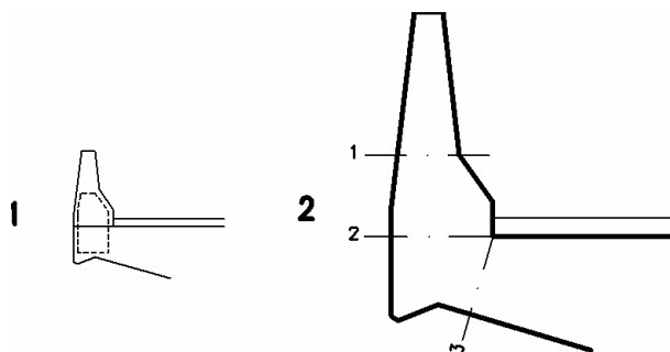
Obrázek 32 – Příklad betonového svodidla „jiného“
