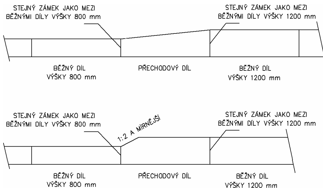
Obrázek 30 – Přechod přímým spojením mezi betonovými svodidly jednoho výrobce
