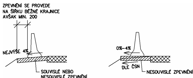
Obrázek 7 – Osazení svodidla v příčném sklonu
