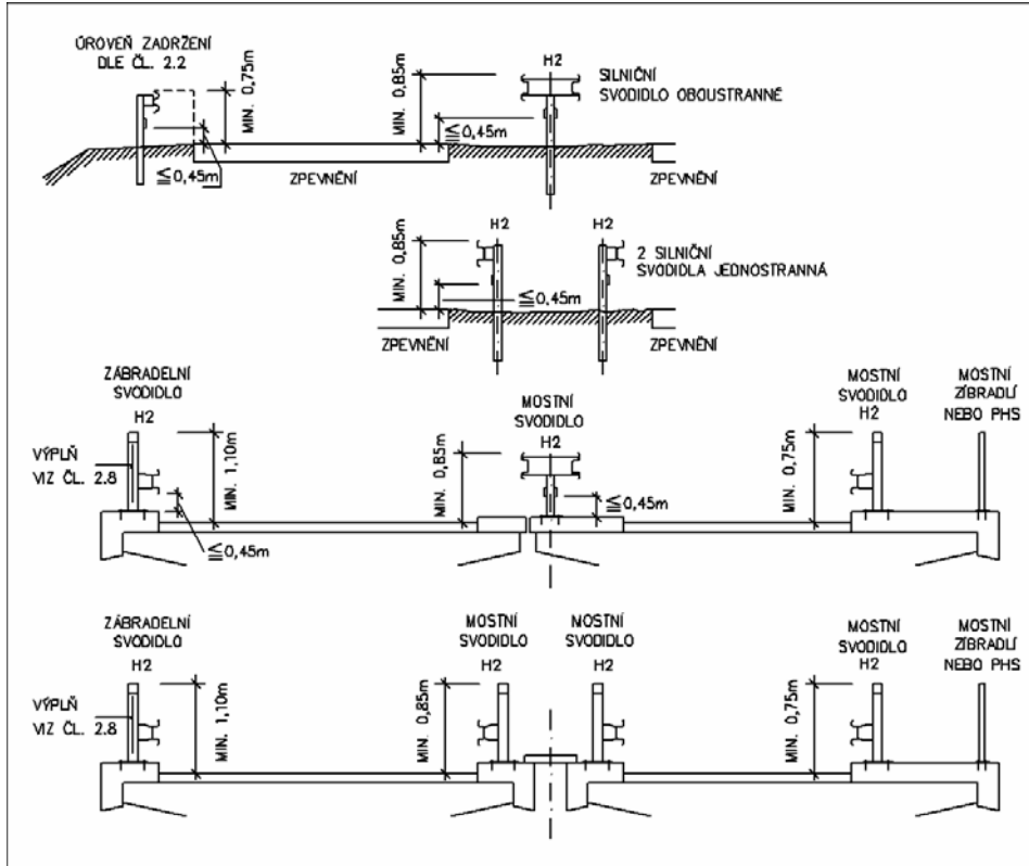
Obrázek 2 – Příklad silničního, mostního a zábradelního svodidla, pokud je v SDP svodidlo úrovně zadržení H2
